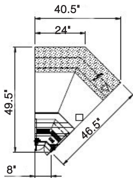
CIF 45°
