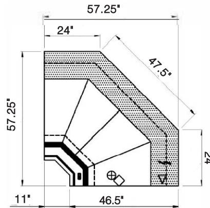
CIF 90°
